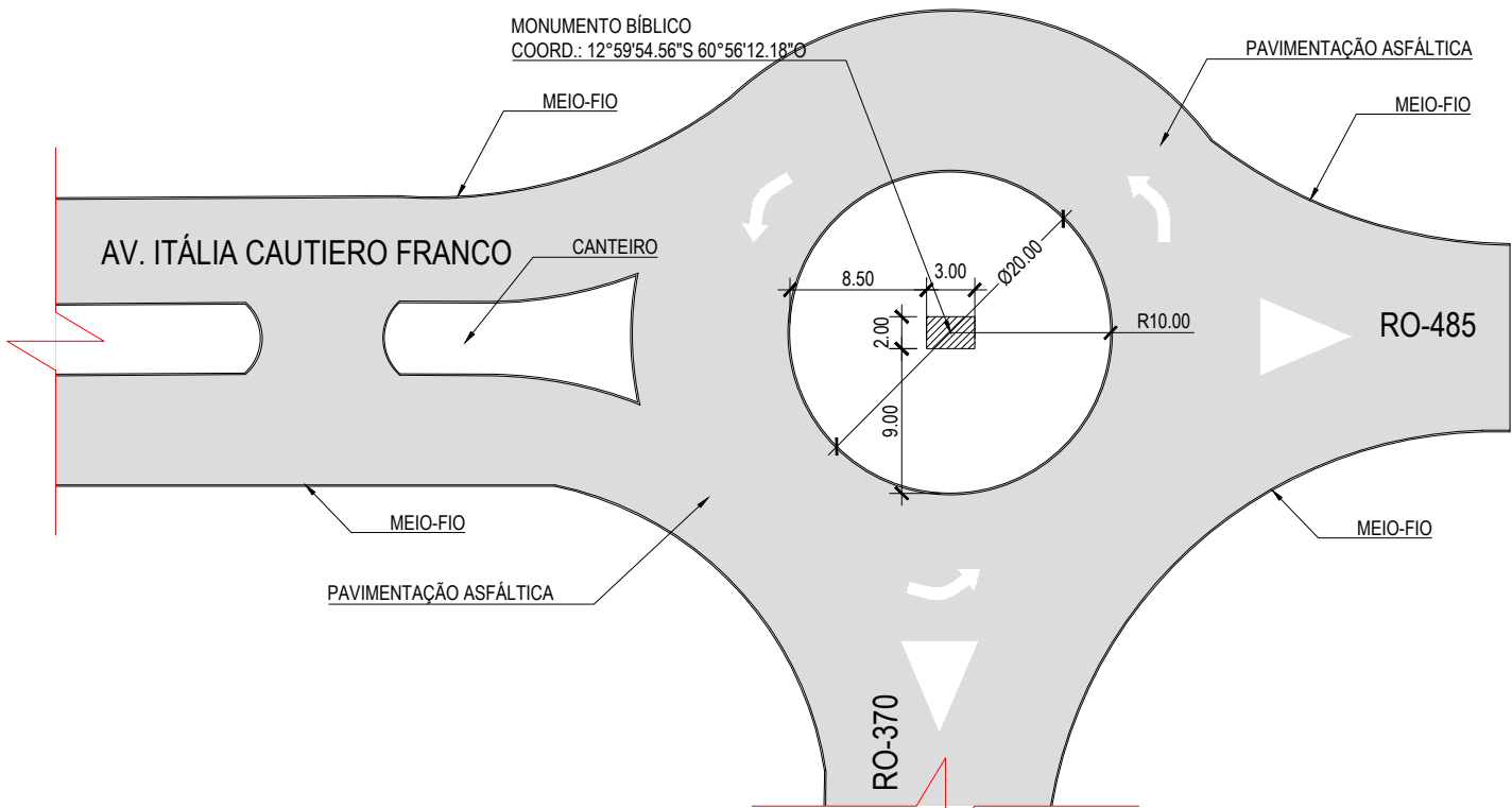
02 IMPLANTAÇÃO - MONUMENTO BÍBLICO ESCALA: 1/500
